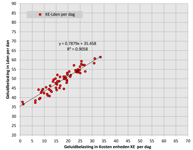
KE-Lden per dag vliegbasis Leeuwarden meetpunt 11 menaldum mei-juni-juli-aug 2022
