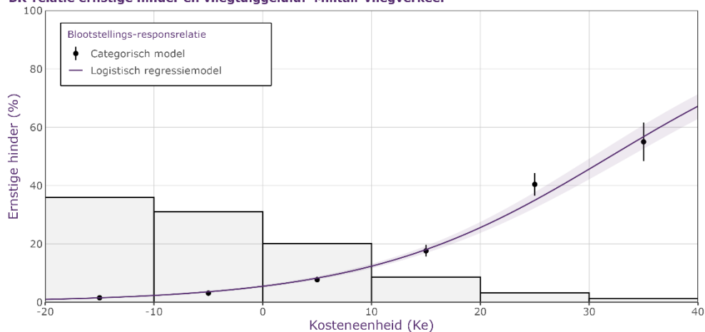
Figuur B2.1 Blootstelling-responsrelatie (BR-relatie) tussen ernstige hinder en blootstelling aan vliegtuiggeluid (Kosteneenheid, berekend met NRM binnen de studiegebieden van militaire luchthavens.
