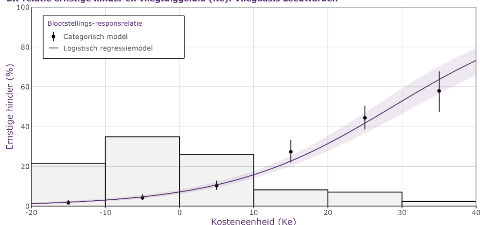
Figuur 4.13 Blootstelling-responsrelatie (BR-relatie) tussen ernstige hinder en blootstelling aan vliegtuiggeluid (Kosteneenheid, berekend met Nederlandse Rekenmodel (NRM)) in studiegebied van vliegbasis Leeuwarden.
