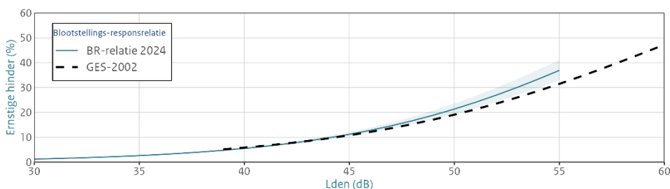
Vergelijking BR-relatie 2024 met GES-2002: Vliegbasis Eindhoven
