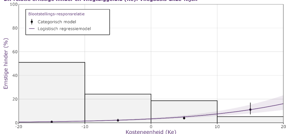
Figuur 4.9 Blootstelling-responsrelatie (BR-relatie) tussen ernstige hinder en blootstelling aan vliegtuiggeluid (Kosteneenheid, berekend met Nederlandse Rekenmodel (NRM)) in studiegebied van vliegbasis Gilze-Rijen.
