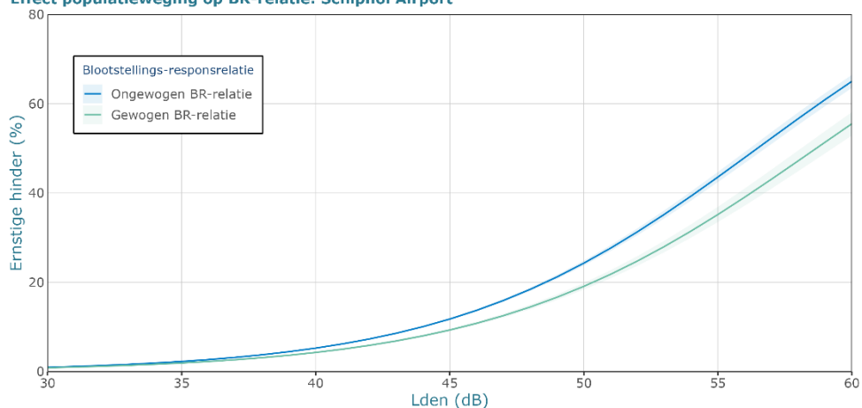
Figuur 5.3 Vergelijking ongewogen en gewogen Blootstelling-responsrelatie (BR-relatie) tussen ernstige hinder en blootstelling aan vliegtuiggeluid ( L_{den} , berekend met Doc29 of Nederlands Rekenmodel (NRM)) rondom Schiphol Airport, Rotterdam The Hague Airport en Vliegbasis Volkel.
