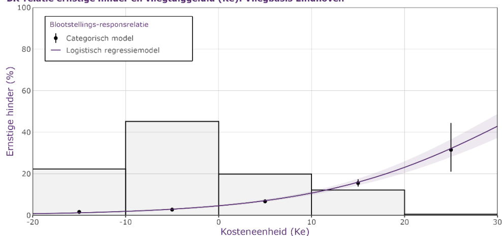
Figuur 4.6 Blootstelling-responsrelatie (BR-relatie) tussen ernstige hinder en blootstelling aan vliegtuiggeluid (Kostenleenheid, berekend met Nederlandse Rekenmodel (NRM)) rondom Vliegbasis Eindhoven.
