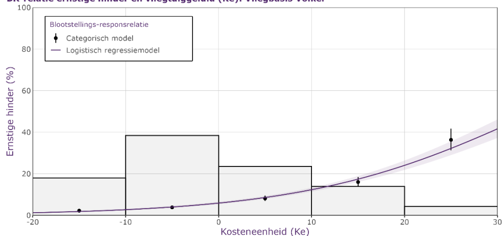
BR-relatie ernstige hinder en vliegtuiggeluid (Ke): Vliegbasis Volkel
