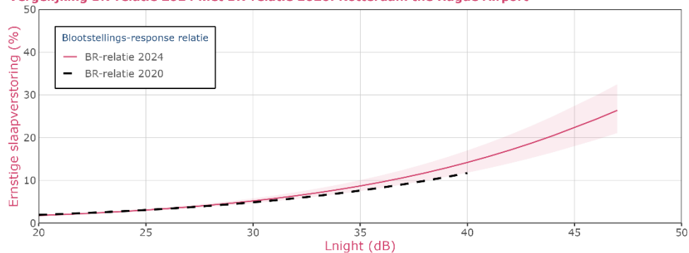
Vergelijking BR-relatie 2024 met BR-relatie 2020: Rotterdam the Hague Airport
