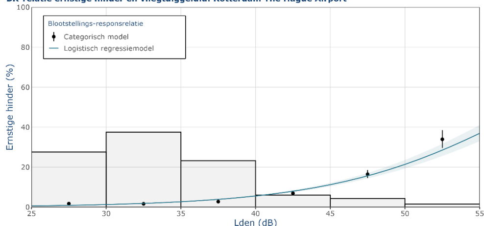
BR-relatie ernstige hinder en vliegtuiggeluid: Rotterdam The Hague Airport
