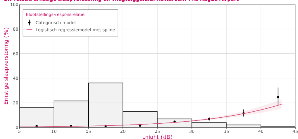
Figuur 4.4 Blootstelling-responsrelatie (BR-relatie) tussen ernstige slaapverstoring en blootstelling aan vliegtuiggeluid ( L_{night} , berekend met Nederlandse Rekenmodel (NRM)) rondom Rotterdam The Hague Airport.
