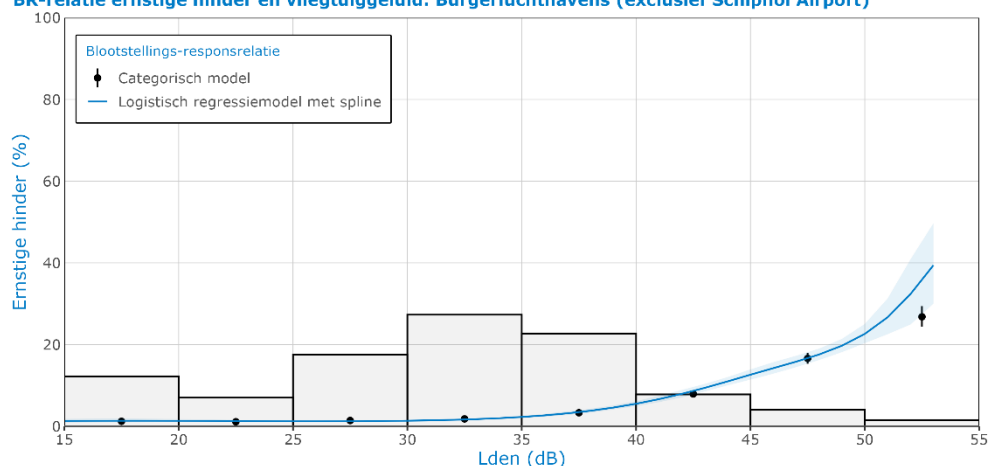
BR-relatie ernstige hinder en vliegtuiggeluid: Burgerluchthavens (exclusief Schiphol Airport)
