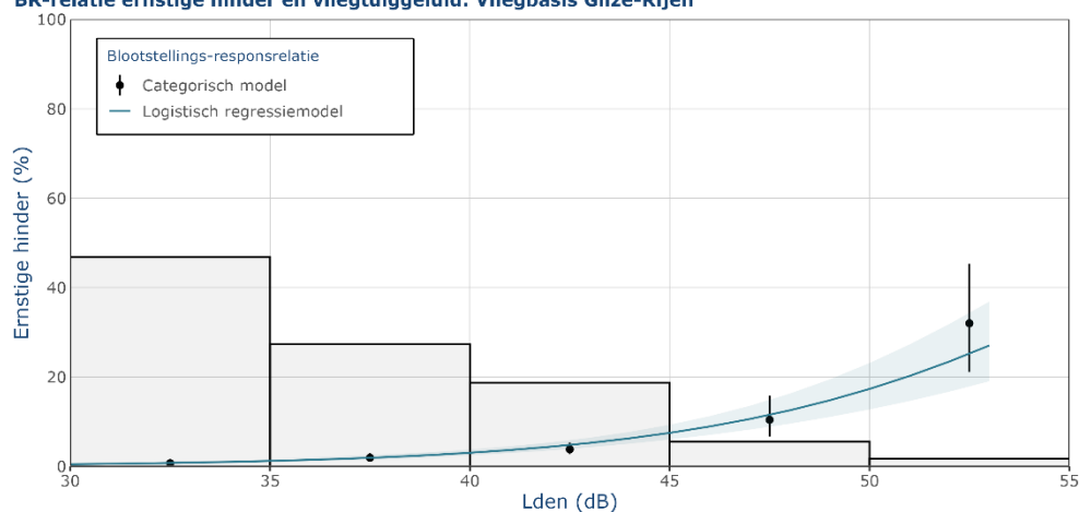
BR-relatie ernstige hinder en vliegtuiggeluid: Vliegbasis Gilze-Rijen
