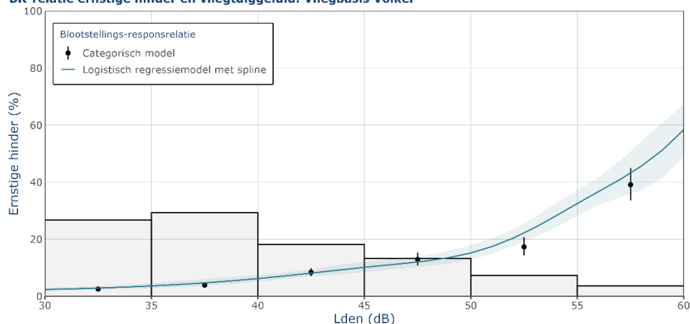
Figuur 4.10 Blootstelling-responsrelatie (BR-relatie) tussen ernstige hinder en blootstelling aan vliegtuiggeluid ( L_{den} , berekend met Nederlandse Rekenmodel (NRM)) in studiegebied van Vliegbasis Volkel.
