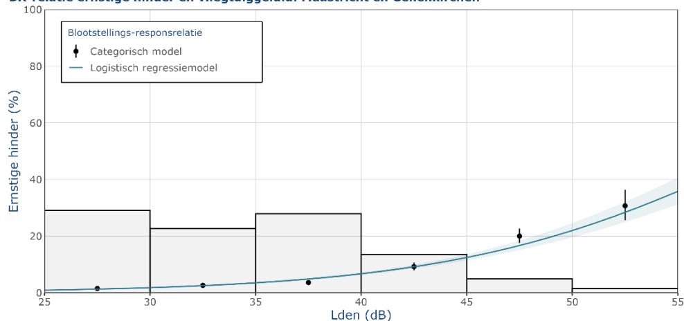
BR-relatie ernstige hinder en vliegtuiggeluid: Maastricht en Geilenkirchen
