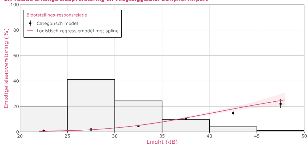
Figuur 4.2 Blootstelling-responsrelatie (BR-relatie) tussen ernstige slaapverstoring en blootstelling aan vliegtuiggeluid ( L_{night} , berekend met het Doc29- rekenmodel) rondom Schiphol Airport.
