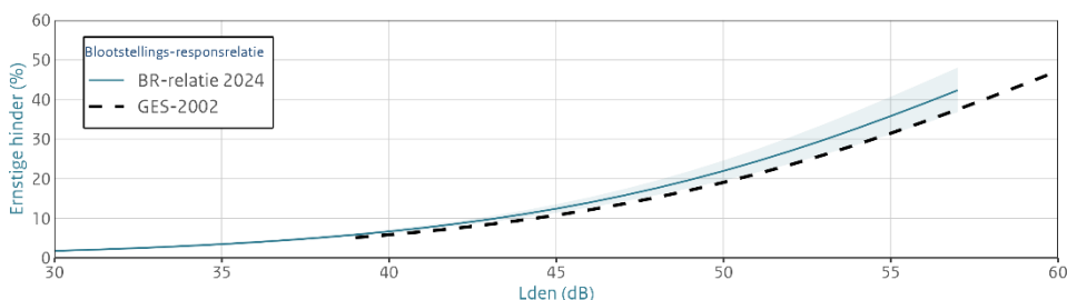
Vergelijking BR-relatie 2024 met GES-2002: Maastricht & Geilenkirchen
