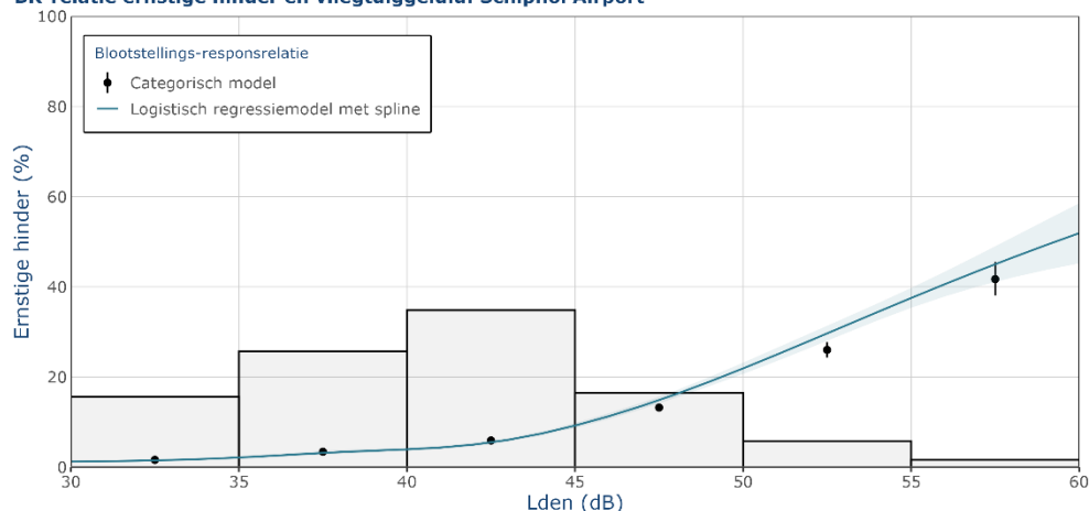
BR-relatie ernstige hinder en vliegtuiggeluid: Schiphol Airport
