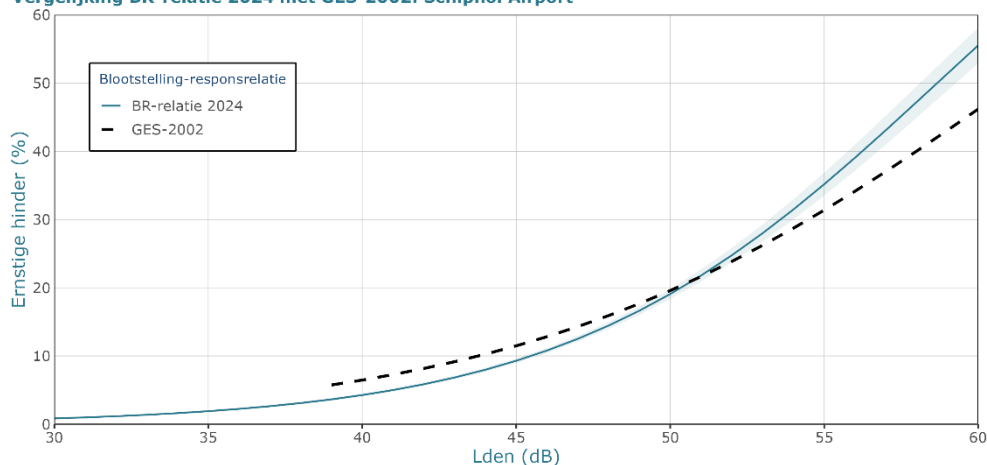
Figuur 4.18 Blootstelling-responsrelatie (BR-relatie) tussen ernstige hinder en blootstelling aan vliegtuiggeluid ( L_{den} , berekend met het Doc29-rekenmodel) rondom Schiphol Airport.
