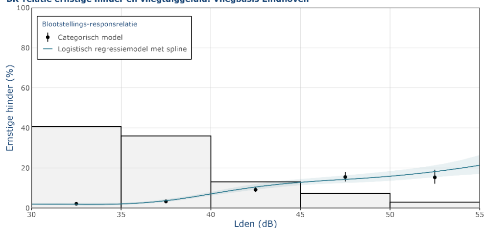
Figuur 4.5 Blootstelling-responsrelatie (BR-relatie) tussen ernstige hinder en blootstelling aan vliegtuiggeluid ( L_{den} ), berekend met Nederlandse Rekenmodel (NRM)) in het studiegebied rondom Vliegbasis Eindhoven.
